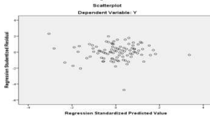
Gambar 7 Hasil Uji Heteroskedastisitas
