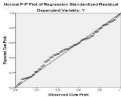
Gambar 6 Pengujian Normalitas
